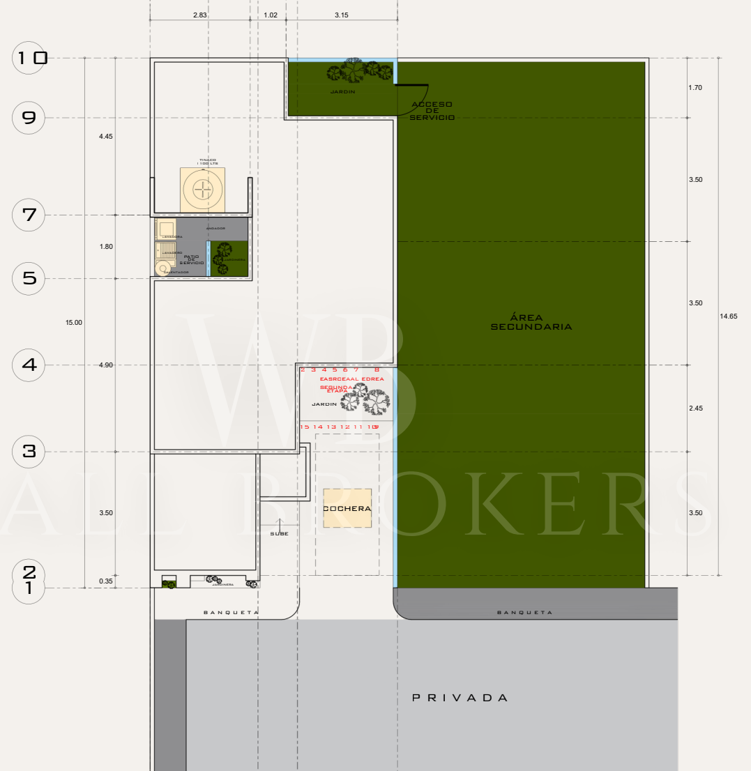
PLANTA AZOTEAS DISTRIBUCION ESD: 1:75
